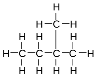
Kekule
